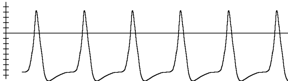
Figura 6: Tren de potenciales de acción.
