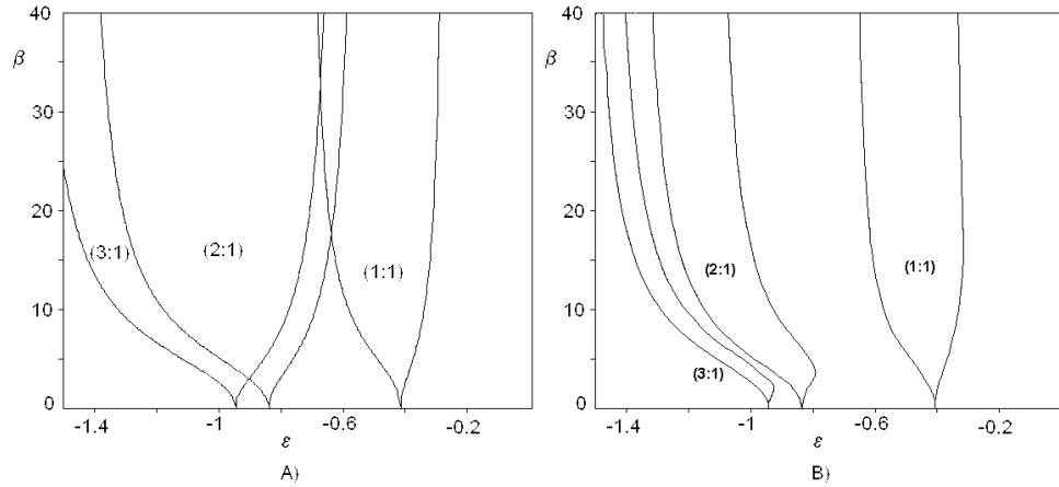
Figura 48: Fronteras de las lenguas de Arnold del modelo de Coombes y Bressloff. Los parámetros \tau y I_0 permanecen constantes en \tau = 1 y I_0 = 2 . A) Diagrama erróneo. Se determinaron las regiones de sincronización determinando si los parámetros de las fronteras de las lenguas determinan soluciones al sistema (26) y además cumplen la condición (28). B) Se efectuó un procedimiento similar, pero determinando si los parámetros dan lugar a órbitas sincronizadas utilizando el algoritmo proporcionado por Carrillo, Ongay y Guzmán.
