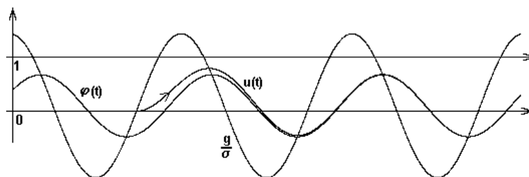
Figura 24: Ilustración de la relación entre la curva de extremos \frac{q(t)}{\sigma} y el atractor periódico \varphi(t) . \sigma = 3 , S = 0.3 , H = 4 .
