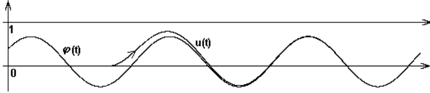
Figura 23: Ilustración de que \max \varphi(t) \leq 1 y \min \varphi(t) \leq 0 no implican que \emptyset \neq D_a \neq \mathbb{R} . \sigma = 3 , S = 0.3 , H = 4 .
