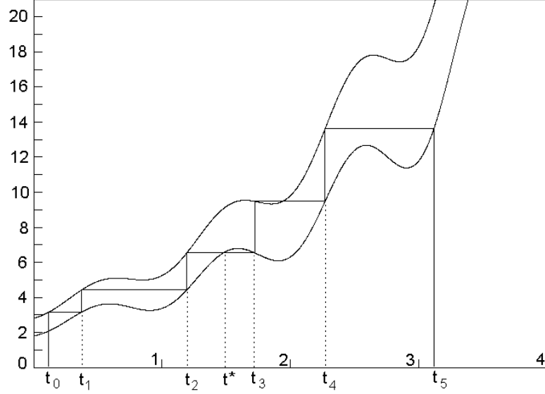
Figura 45: Solución de un sistema de ecuaciones de la forma indicada por (26), que muestra una órbita periódica espuria. Se buscó una órbita sincronizada con sincronización (q : p) = (5 : 3) , con valores de los parámetros \tau = 1.6 , I_0 = 2 , \varepsilon = 2.5 . Los primeros 5 elementos de la órbita son t_0 = 0.11887512 , t_1 = 0.37394849 , t_2 = 1.19351461 , t_3 = 1.72429478 , t_4 = 2.27117296 . Como era de esperarse, t_5 = 3.11887512 = t_0 + p = t_0 + 3 . t^* denota el tiempo real de disparo y t_3 el tiempo erróneo.
