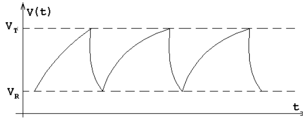
Figura 1: Oscilaciones de diente de sierra.
