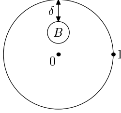
Figura 3.2: La distancia del disco B a |z| = 1 .
